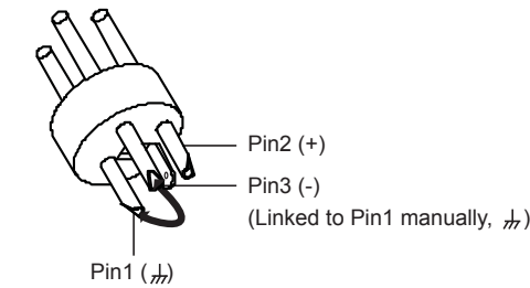
XLR, unsymmetrisch
