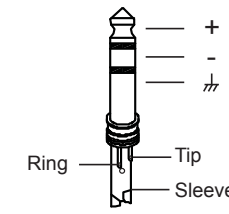
Stereoklinke, symmetrisch
