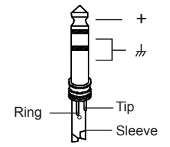
Stereoklinke, unsymmetrisch
